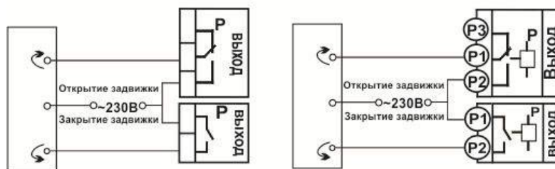
Подключение электрозадвижки
